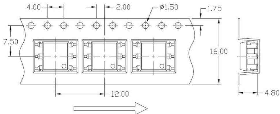
图 5 编带包装示意图 Figure 5- Taping Packing Schematic
