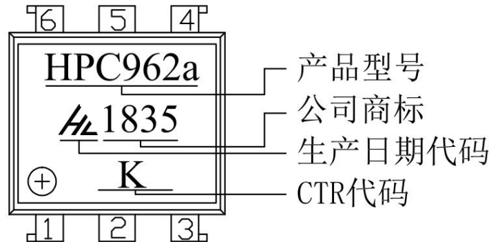
图 4 产品印章 Figure 4- Marking
