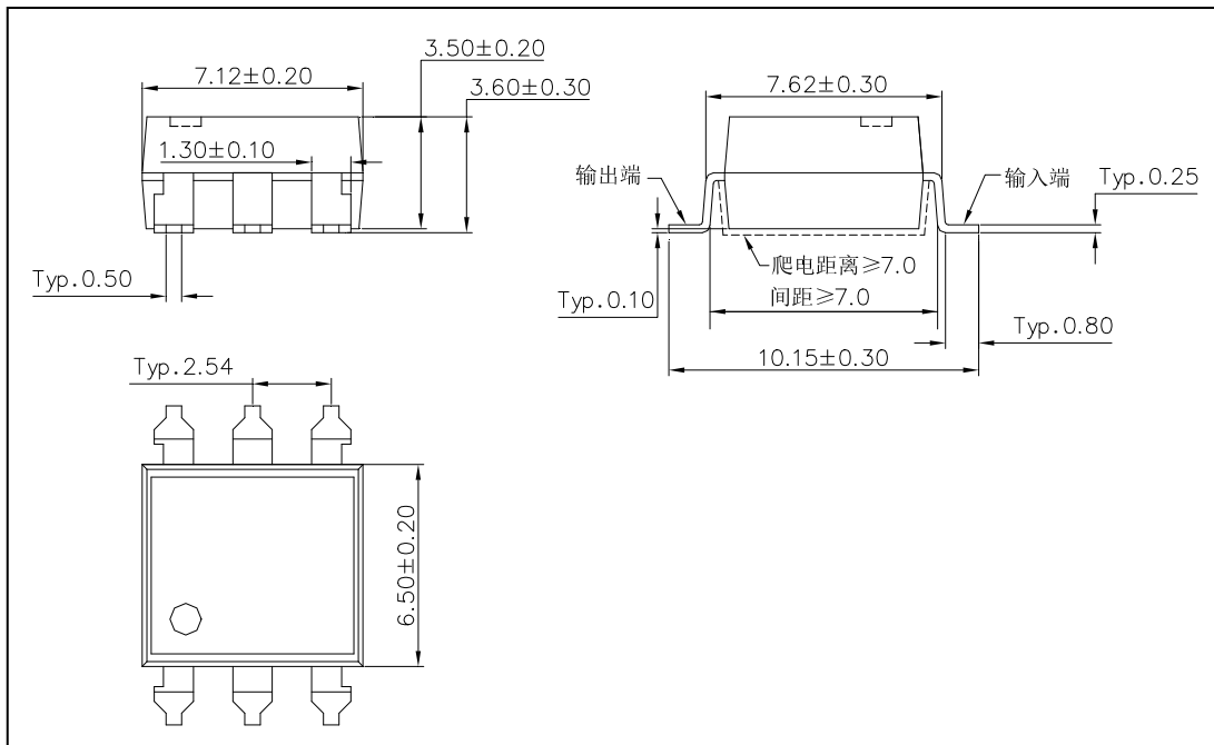
图 3 HPC962Ka-2 外形尺寸 Figure 3- The dimensions of HPC962Ka-2
