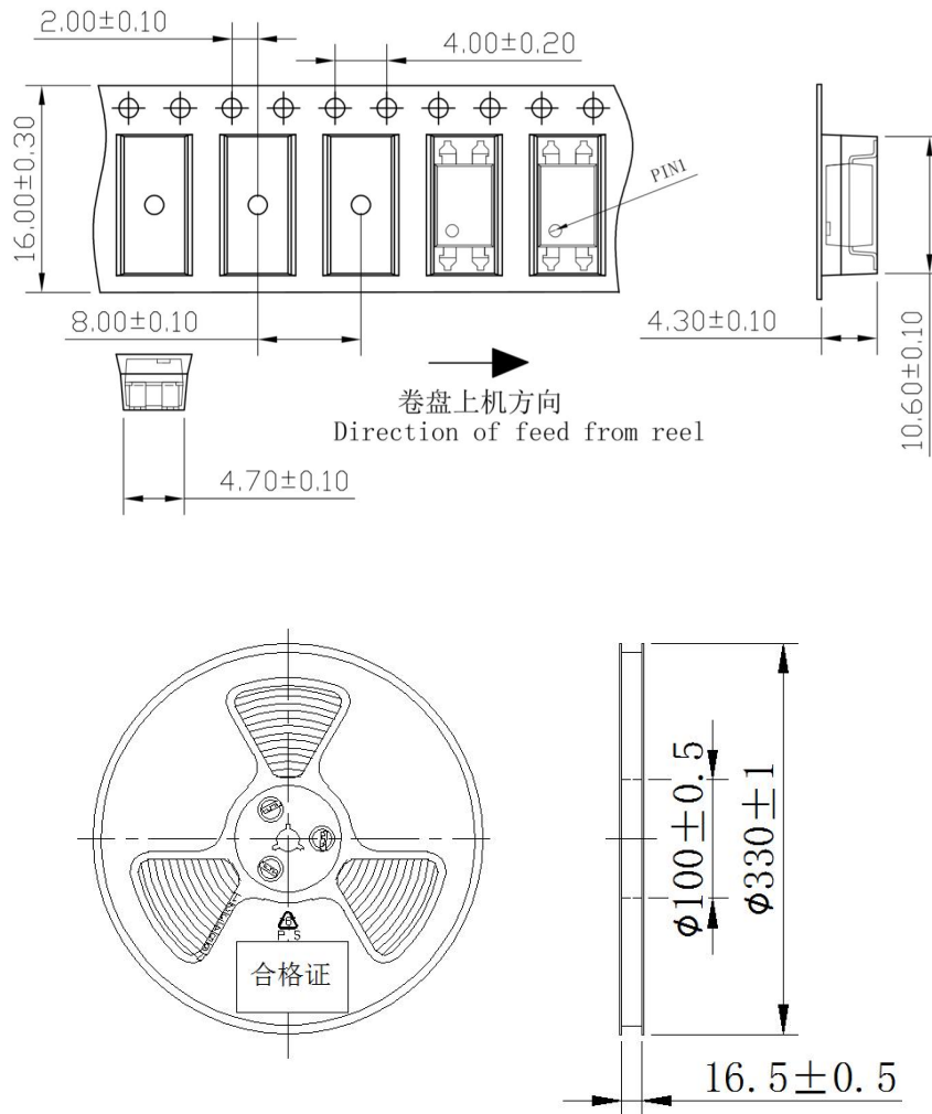
图 8 编带包装示意图
