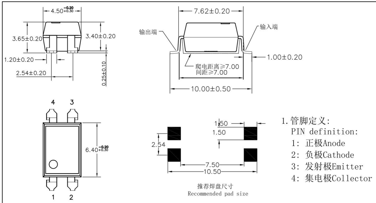
图 5 HPC817×h-2 外形尺寸
