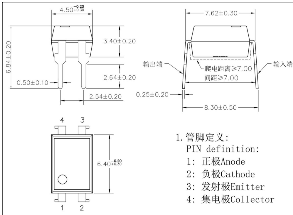
图 4 HPC817×h 外形尺寸
