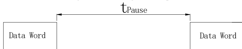
图 3 信号间隔时间 Figure3 Date Pause Time
