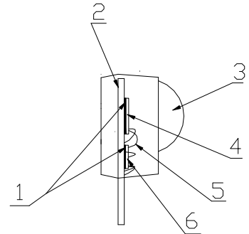
图 7 结构和材料
