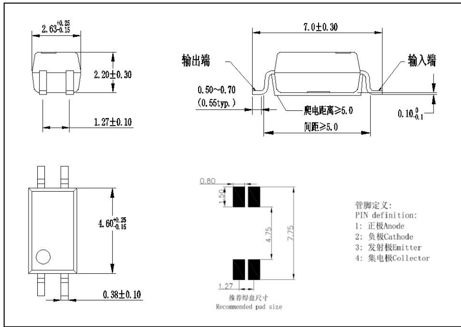
图 4 HPC214× 外形尺寸 Figure 4- The dimensions of HPC214×
