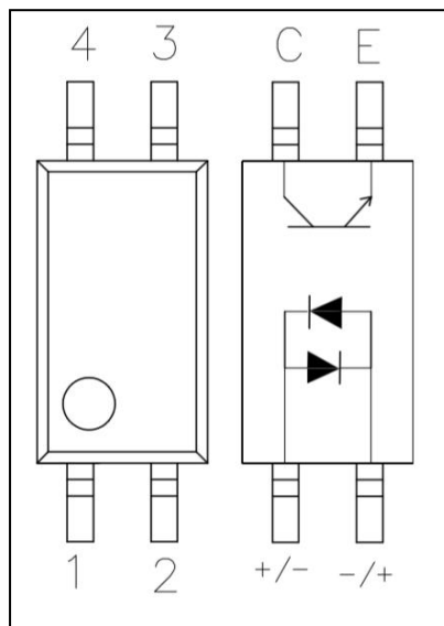
图 3 电原理图 Figure 3-Schematic
